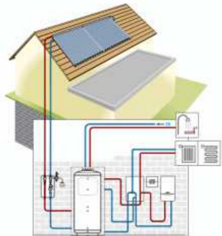
Solární systém Vaillant na podporu vytápění a k ohřevu teplé vody s kombinovaným zásobníkem auroSTOR VPS SC 700
