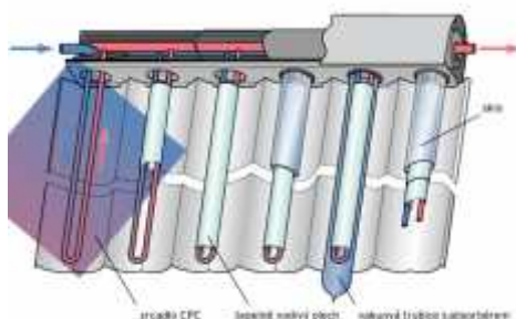
Průběh proudění a konstrukce kolektoru auroTHERM exclusiv VTK 570/2
